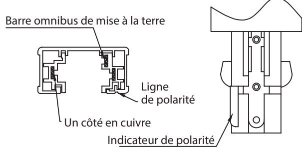
FIG. 2 Polarité standard
